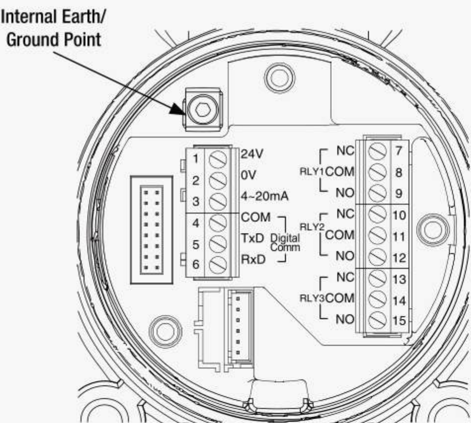
Terminal Module
